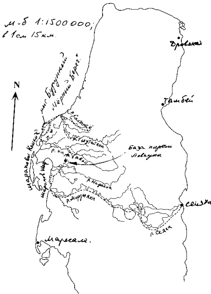
Рис. 1. Карта-схема маршрутов на Ямале
